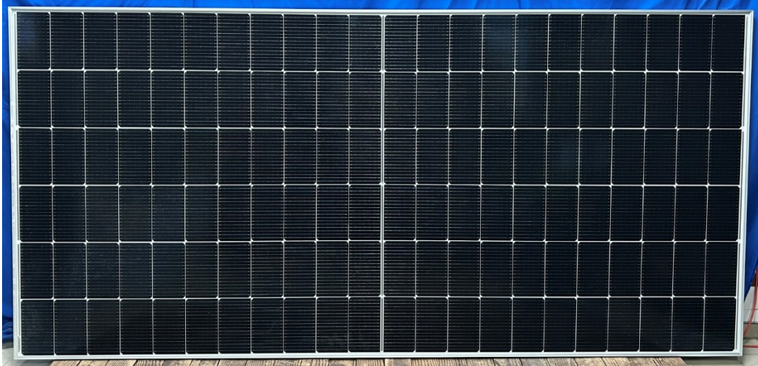
Fig. 1: Front view of module type ERA-RC-66HC610M Fig. 1: Vista frontal do tipo de módulo ERA-RC-66HC610M
